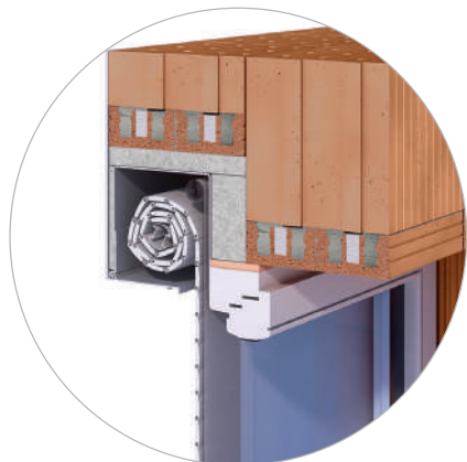
Unterputzkasten
