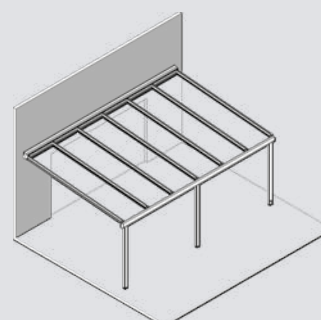
B3 Bündig, 3. Steher
